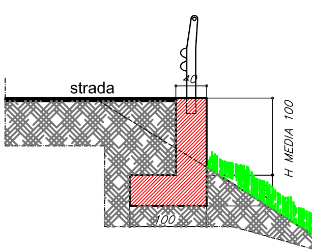
SEZIONE 6
