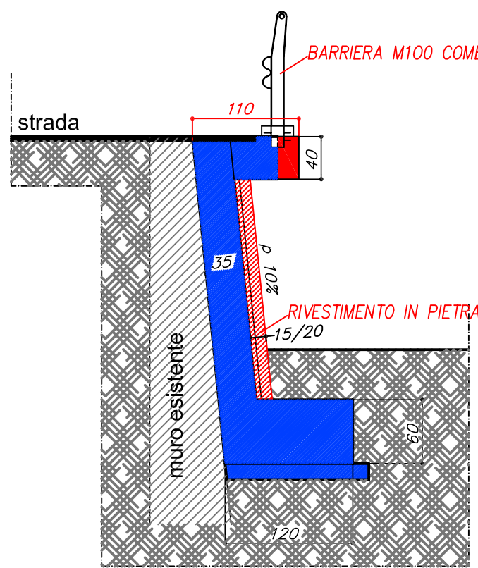
SEZIONE 2
