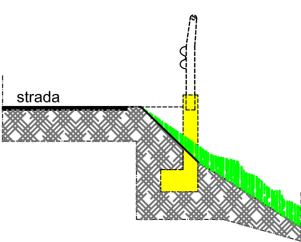
SEZIONE 8 da non realizzare
