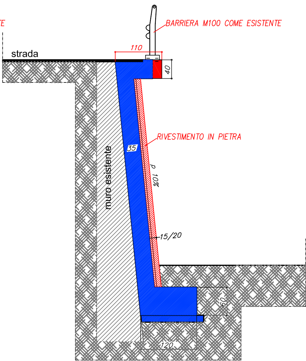
SEZIONE 3
