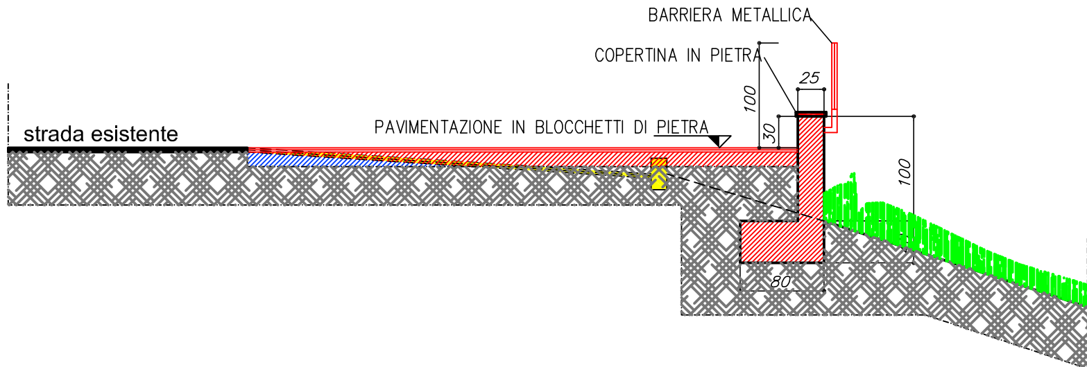
SEZIONE 7
