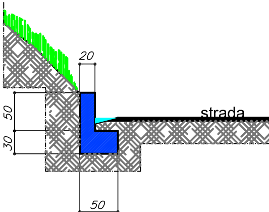
SEZIONE 5
