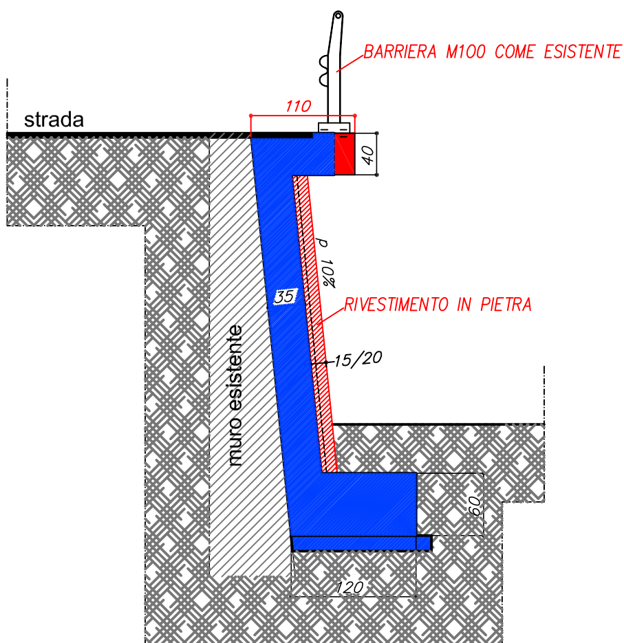
SEZIONE 4
